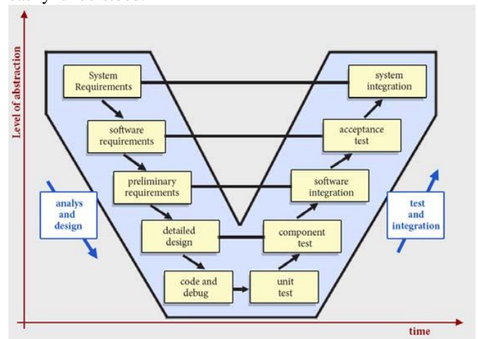
Fig. 5 V-Model [3]
